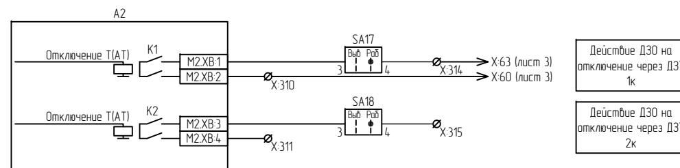
Выходные цепи А2
