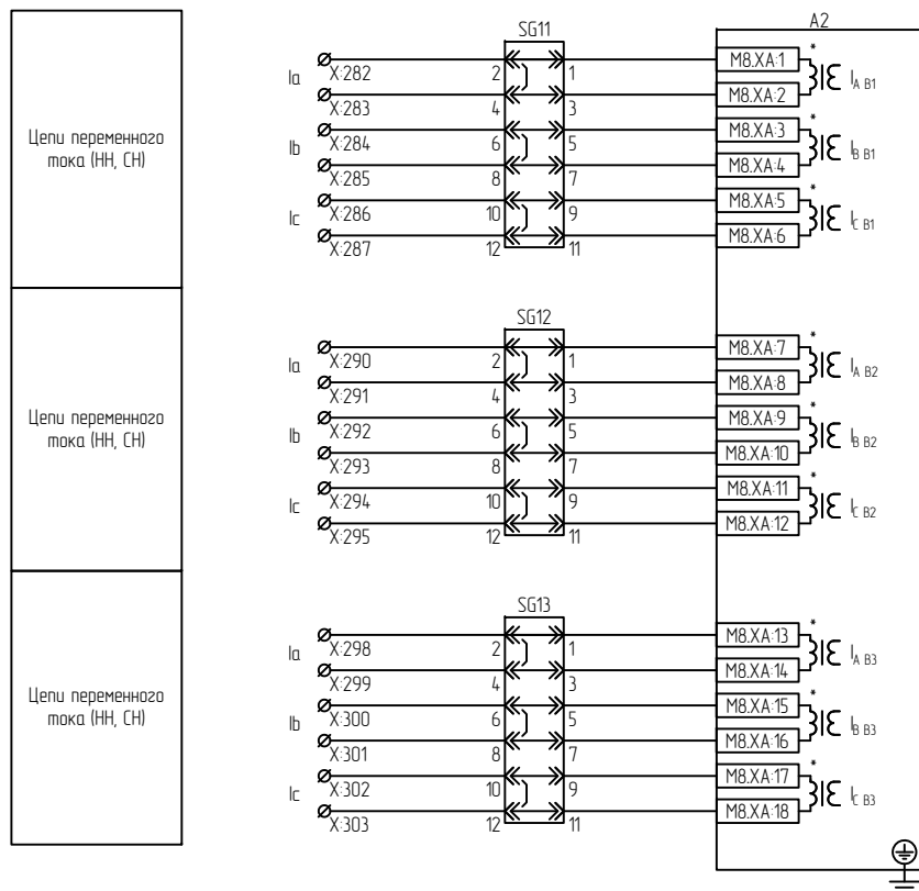
Цепи переменного тока и напряжения А2
